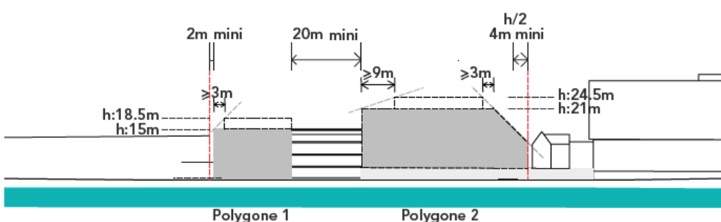
Limites de hauteur côté quai, retrait des attiques, elevation sud-ouest / nord-est
